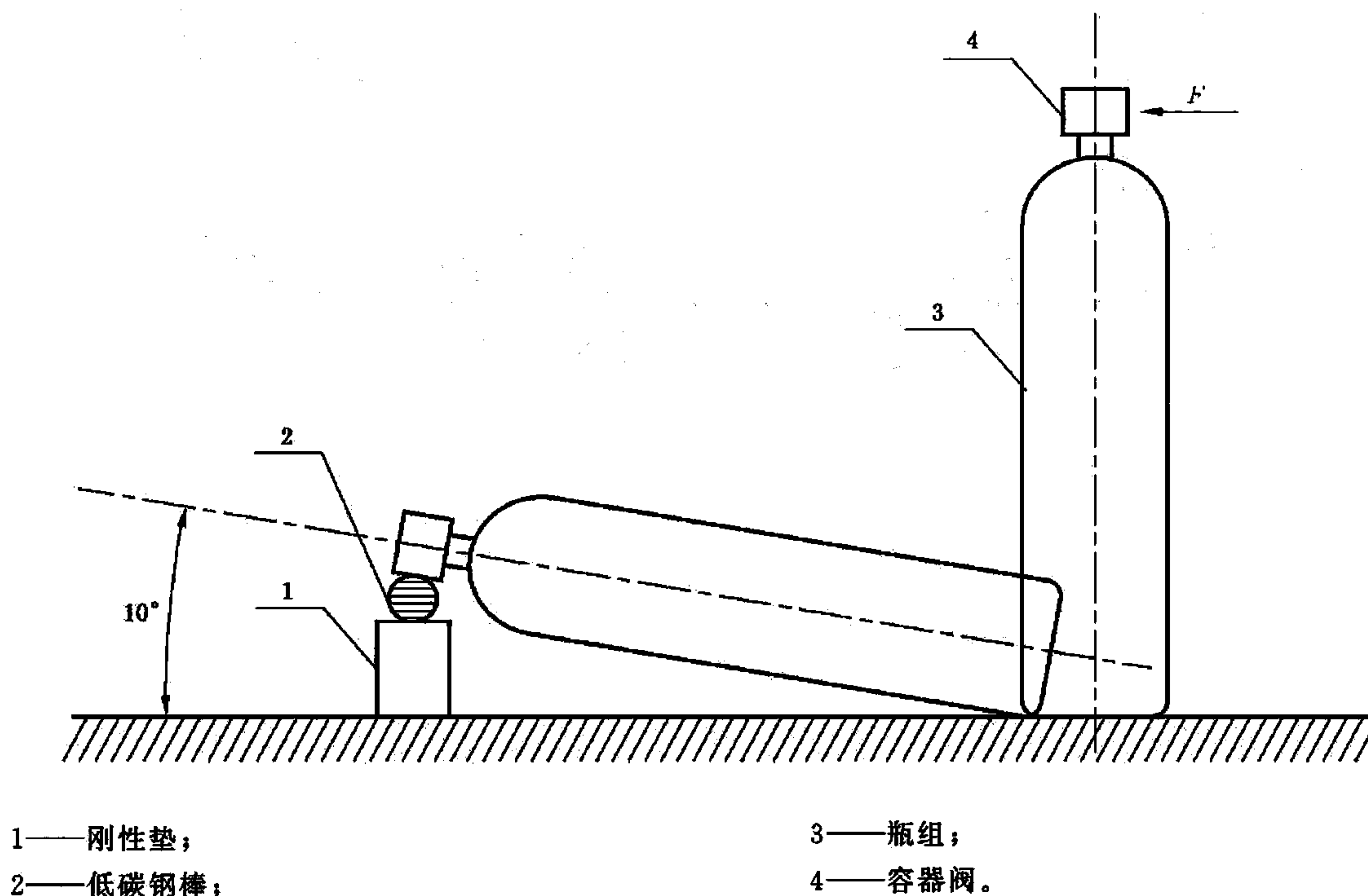
图 2 倾倒冲击试验示意图
