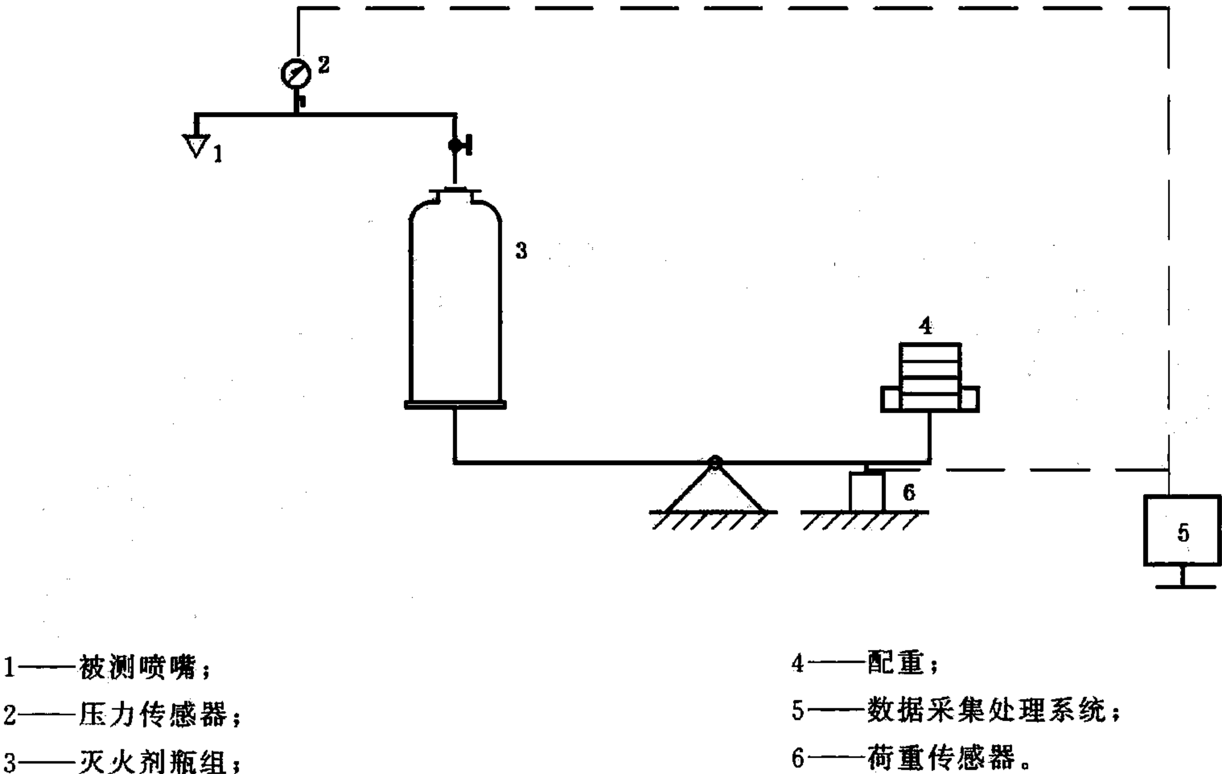
a) 重量平衡方式
